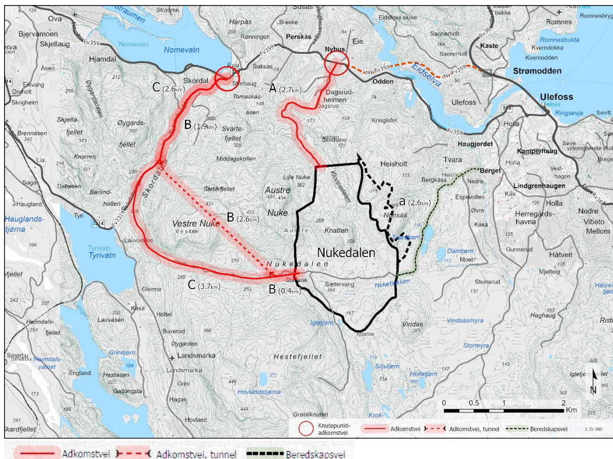
Figur 3.8 Kartet viser avgrensing av Nukedalen-alternativet med mulig adkomstveger / tunnel og knutepunkt til eksisterende veg. I tillegg vises mulige beredskapsveger.
