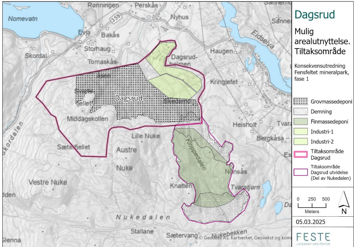
Figur 1: Kartet viser avgrensning av Dagsrud-området med plassering av tiltakene (industriarealer, deponi for fine masser og deponi for grove masser med areal for framtidig industri). Mørkegrå arealer viser plassering av demninger for deponi.
