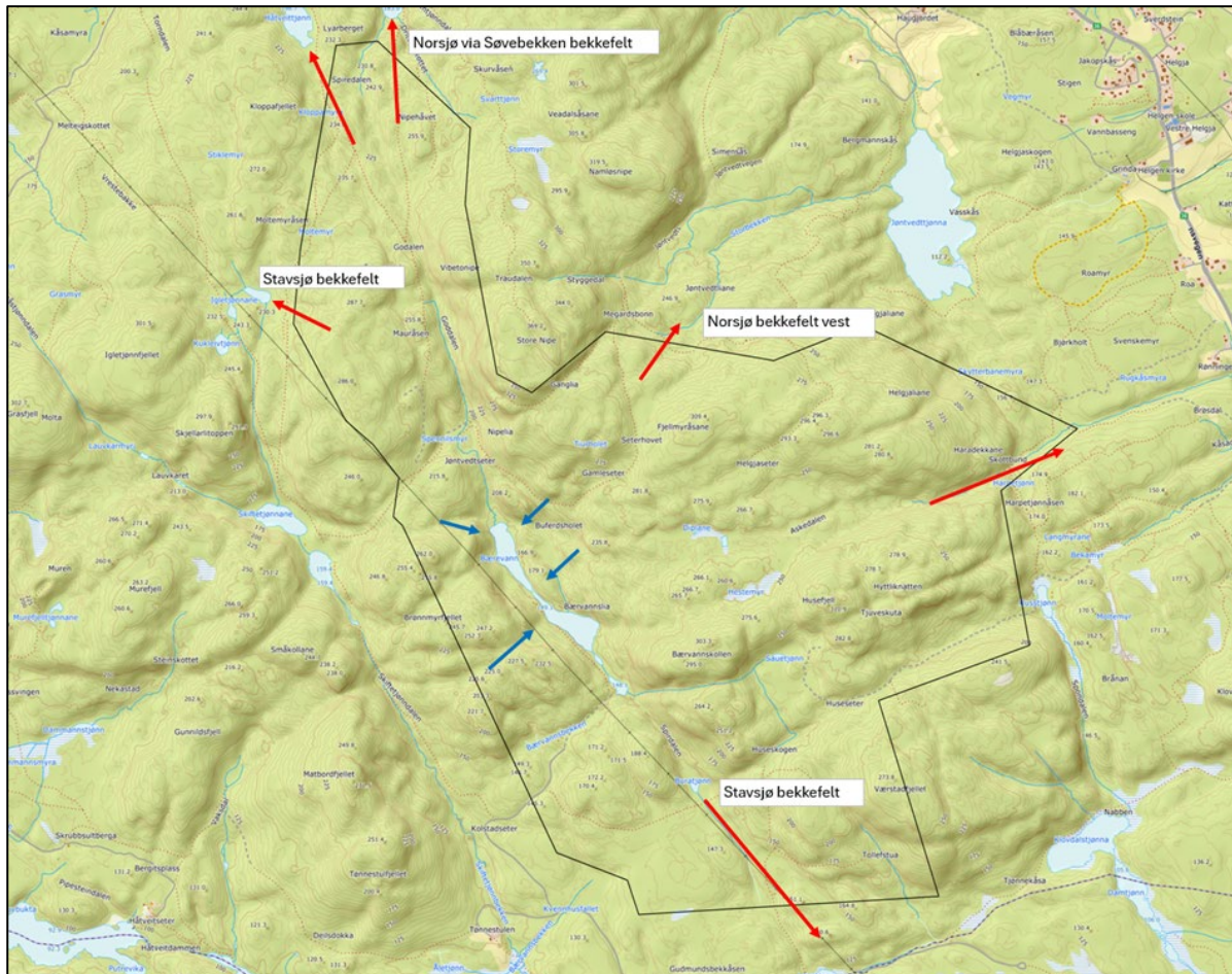
Figur 3.2: Avrenningsmønster Bærevann, utklipp fra Scalgo. Blå pil indikerer vann som renner inn i området, rød pil indikerer vannretning ut av området.
