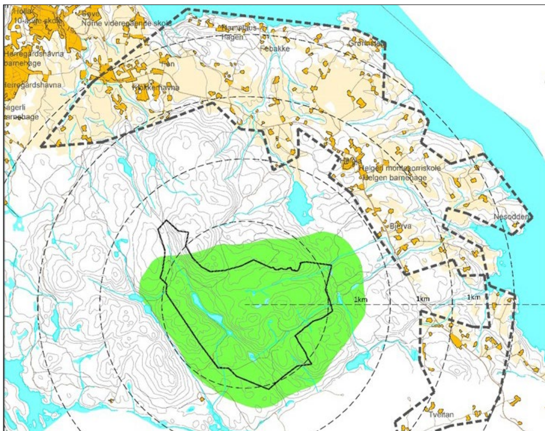
Figur 3.7: Kartet viser støysone-beregninger for "stille områder" beregnet for Bærevann-tiltaket. Det grønne arealet viser støygrensen 50 dBA Lden. Denne viser grenseverdien gjelder for sammenhengende grønnstruktur i tettsteder. Det er derfor valgt å sammenstille denne sonen med utredningsområdet for nærmiljø. Ingen av boligene og deres nærmiljø overskrides av støygrensen 50 dBA Lden ved tiltaket på Bærevann.
